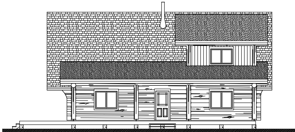
Right Elevation
